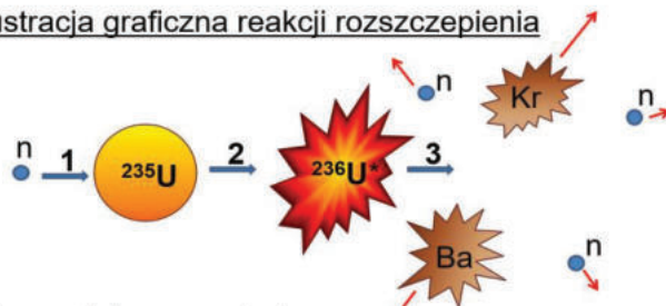
Etapy reakcji rozszczepienia:
